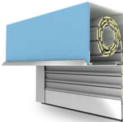
Vorbaurollladen Compacto
