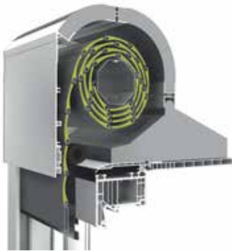
Renoverungsrollladen Cereno
