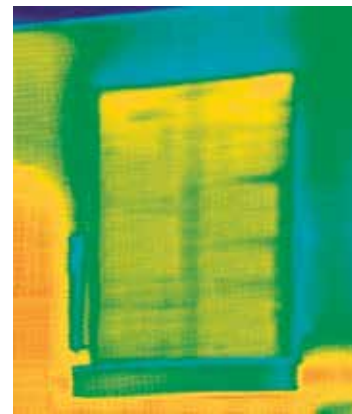
Mit Rollläden, geringer Wärmeverlust
